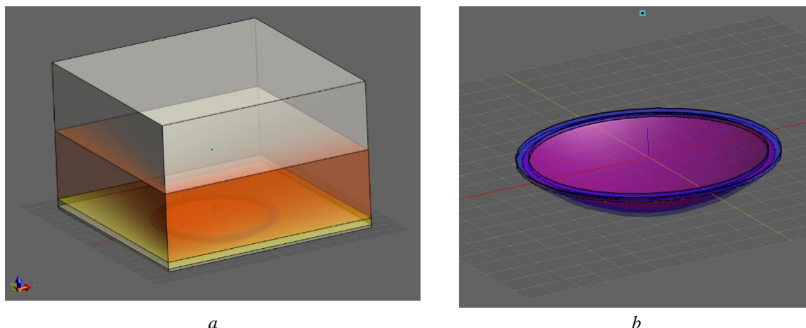
Рис. 1. Модель в пакете Sim4Life: тканей человека (а); одноэлементного фокусирующего излучателя (b) Fig. 1. Model in the Sim4Life: human tissues (a); single element focusing emitter (b)
