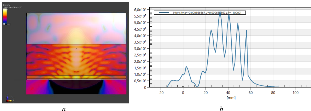
Рис. 3. – Распределение интенсивности в структуре модели при частоте 110 кГц: a – графическое изображение; b – график распределения интенсивности, Вт/м 2
