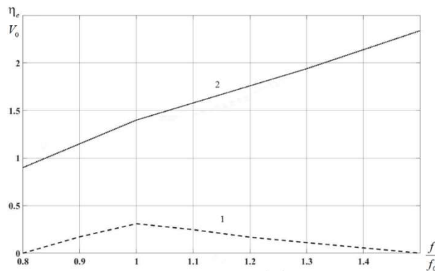
Рис. 4. Перестроечные характеристики генератора: 1 – \eta_e\left(\frac{f}{f_0}\right) ; 2 – V_0[\text{кВ}] = f\left(\frac{f}{f_0}\right)
