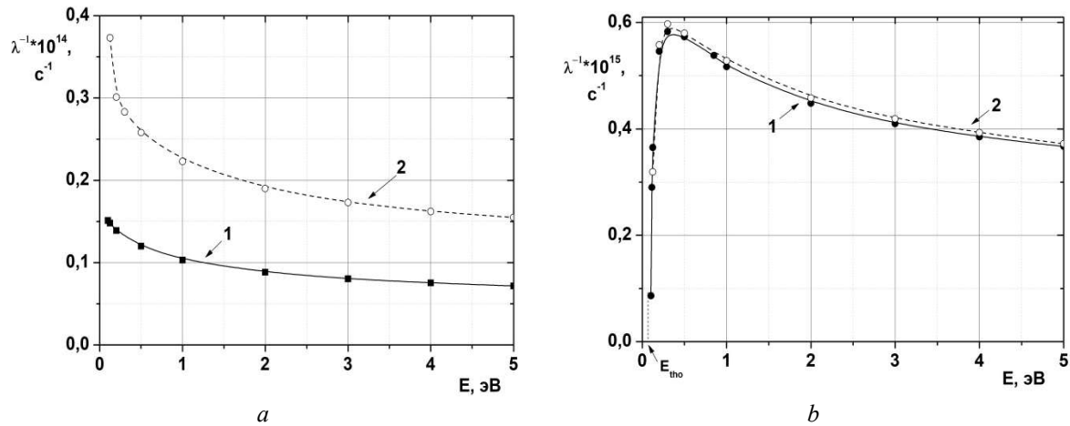
Рис. 2. Зависимости интенсивности рассеяния на полярных оптических фонах при поглощении (а) и испускании (b) фононов от энергии электронов и температуры
