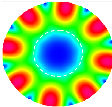
Рис. 4. Поперечное распределение модуля напряженности электромагнитного поля в конце волновода моды H_{41} Fig. 4. Transverse distribution of the electromagnetic field intensity modulus at the end of the waveguide mode H_{41}
