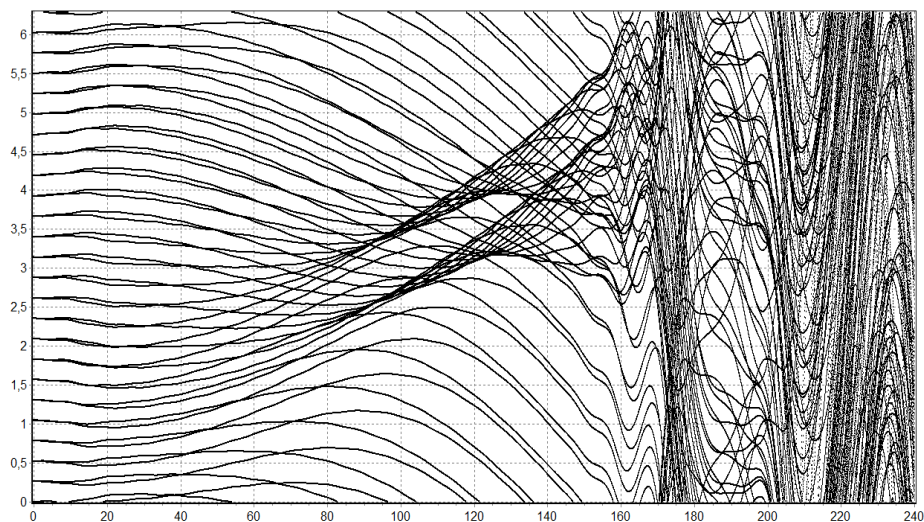
Рис. 5. Фазовые траектории электронов Fig. 5. Phase trajectories of electrons
