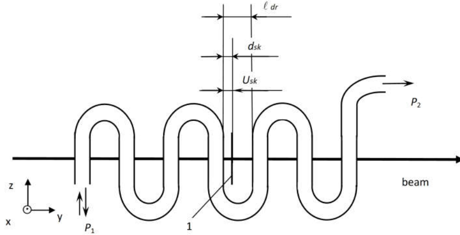
Рис. 1. Схема ЛБВ со скачком потенциала: 1 – пластина, на которую подан потенциал V_{sk} Fig. 1. TWT circuit with a potential jump: 1 – plate to which the potential V_{sk} is applied
