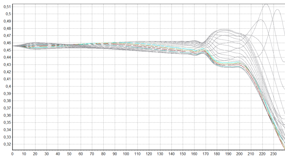
Рис. 6. Поперечные нормированные скорости электронов Fig. 6. The normalized transverse velocity of electrons
