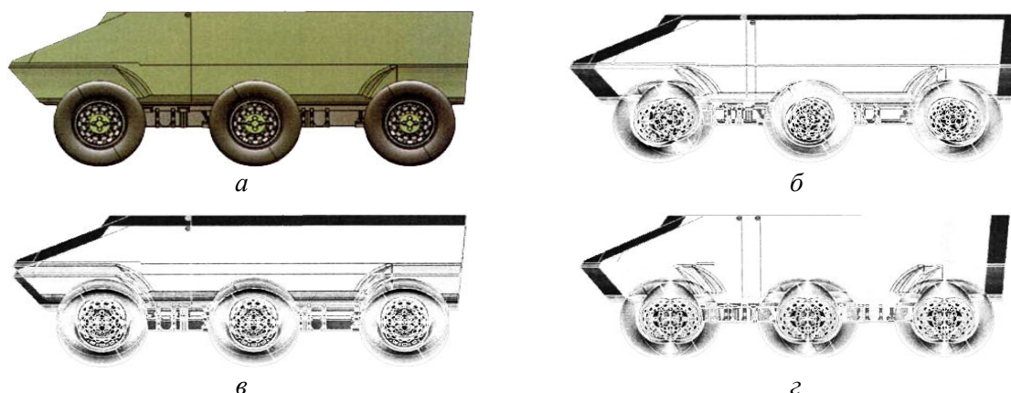
Рис. 1. Межкадровая попиксельная разность |I_{i,j} - I'_{i,j}| для движущегося объекта на однотонном контрастном фоне; а – исходный объект (колесный транспортер); б – приближение объекта; в – движение вверх; г – движение влево
