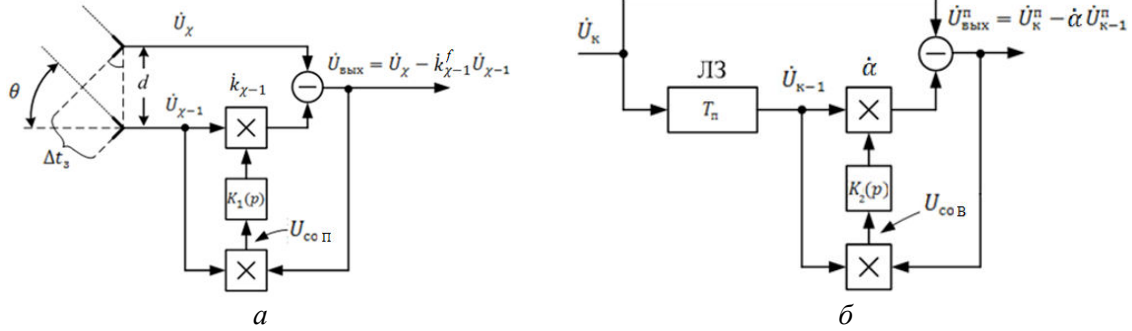
Рис. 1. Модели автокомпенсаторов сигнала помехи: а – междуканальный пространственный фильтр; б – междупериодный временной фильтр
