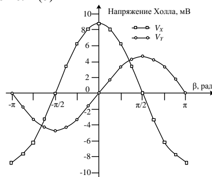
Рис. 4. Зависимости напряжений Холла от угла отклонения beta
