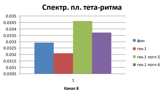
Рис. 4. Гистограммы распределений спектральной плотности мощности тета-ритма электроэнцефалограмм отведений T_4 - A_2 в состояниях, определяемых как режим 1, режим 2, режим 3, режим 4
