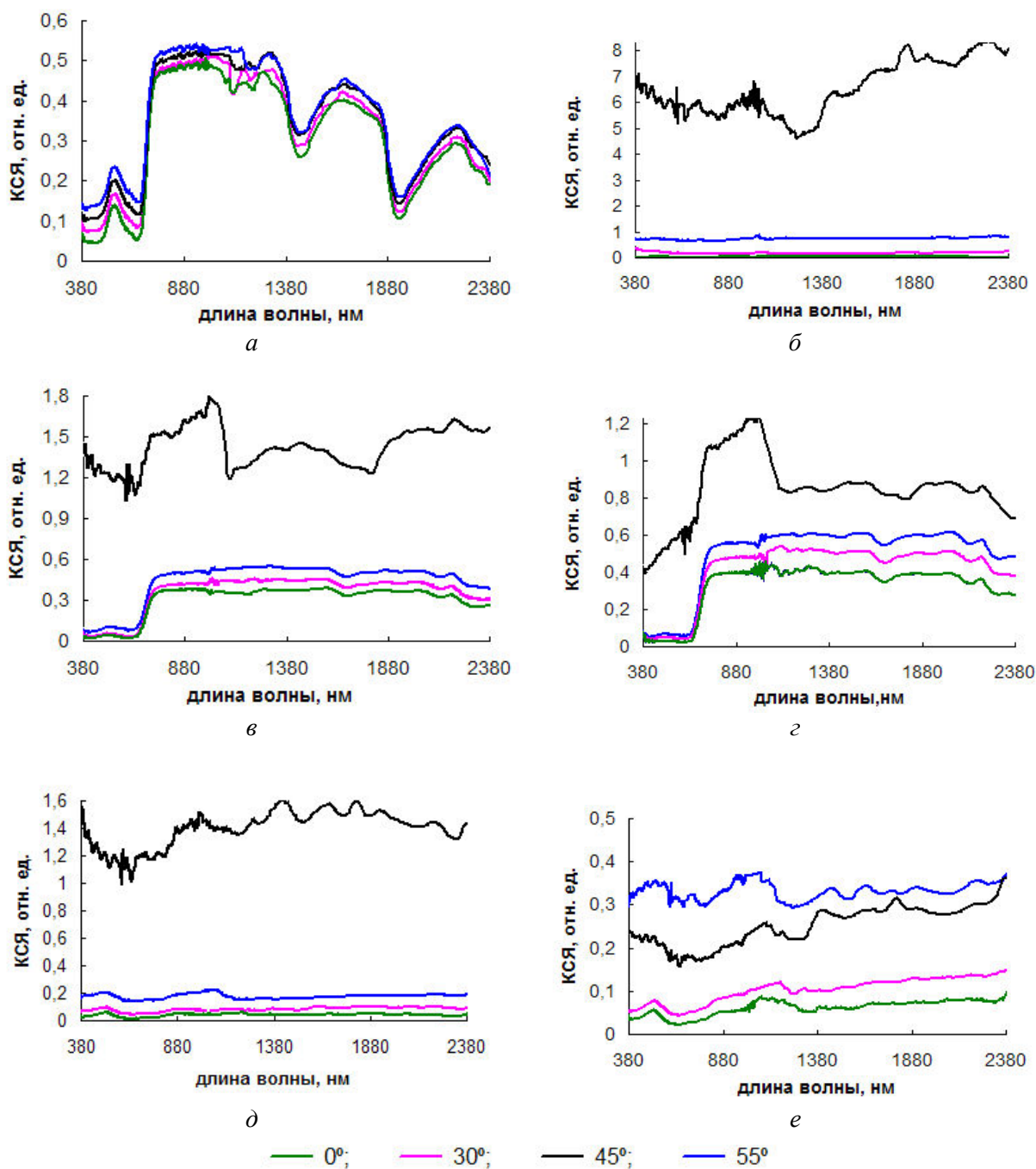
Рис.2. Распределение КСЯ при углах наблюдения 0°, 30°, 45°, 55° для: a – листа растительности; б – пластины окрашенного в зеленый цвет металла; в – образца металла и сетки 1; г – образца металла и сетки 2; д – образца металла и сетки 3; е – образца металла и сетки 4
