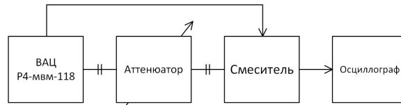
Рис. 2. Схема эксперимента
