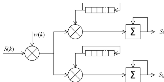
Рис. 1. Схема, реализующая квадратурное разложение и накопление измерительного сигнала
