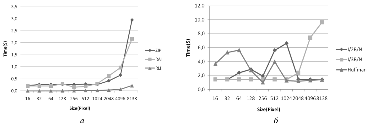
Рис. 5. Зависимости времени кодирования изображений от их размера: а – для алгоритмов Zip, Rar, RLE и его предложенных модификаций в операционной системе Windows 7; б – для алгоритмов Хаффмана, I/2B/N и I/3B/N в среде Matlab 2012
