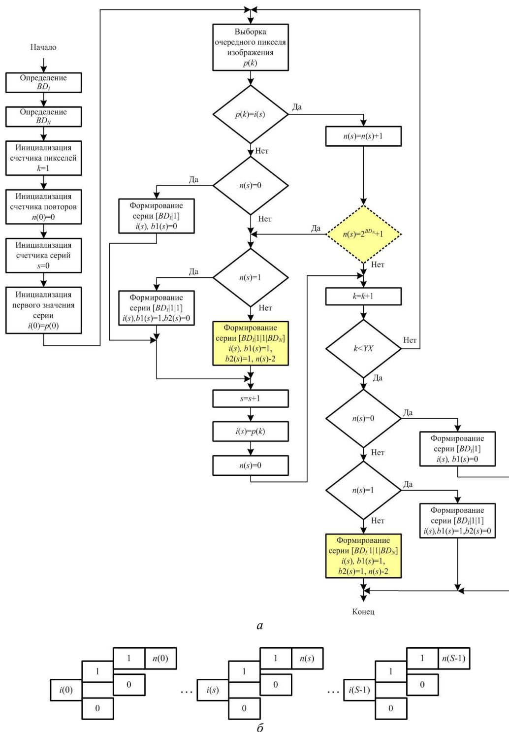
Рис. 2. Модифицированное I/2B/N кодирование длин серий: а – алгоритм I/2B/N кодирования длин серий; б – структура закодированных данных по алгоритму I/2B/N
