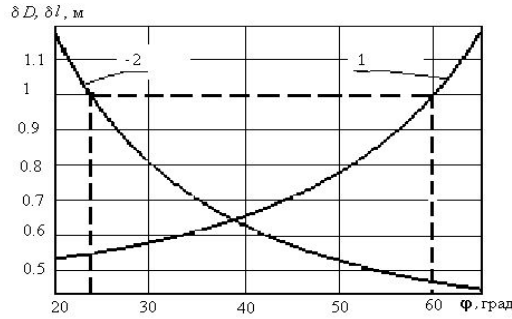
Рис. 3. Зависимость изменения разрешающей способности по горизонтальной дальности \delta D (зависимость 1) и азимуту \delta l (зависимость 2) от угла \varphi
