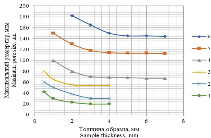
Рис. 3. Распределение максимальных размеров пор по толщине образцов, полученных из порошков различного гранулометрического состава с применением вибрации (размер частиц: 1 – (–0,063 ... +0,04); 2 – (–0,1 ... +0,063); 3 – (–0,16 ... +0,1); 4 – (–0,2 ... +0,16); 5 – (–0,315 ... +0,2); 6 – (–0,4 ... +0,315) мм)
