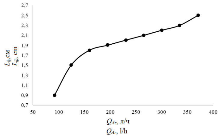
Рис. 2. Зависимость длины факела плазменной струи от расхода плазмобразующего газа Fig. 2. Dependence of the plasma torch length on the plasma-forming gas flow rate
