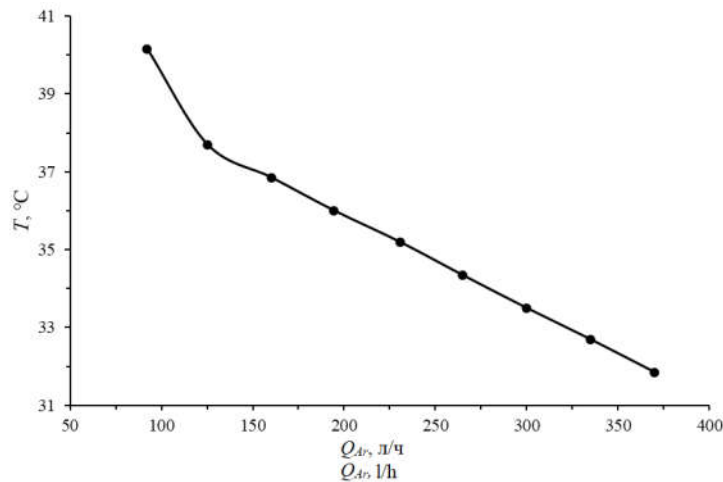
Рис. 3. Зависимость температуры объекта обработки в плазменной струе от изменения расхода газа Fig. 3. Dependence of the plasma treated object temperature on the gas flow rate.
