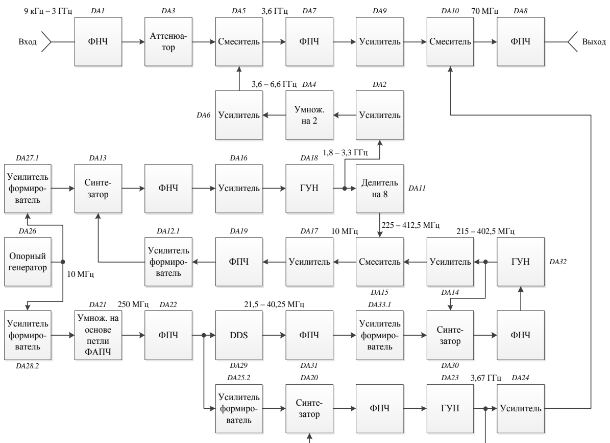
Рис. 1. Блок-схема СВЧ анализатора спектра с использованием двухпетлевой системы ФАПЧ
