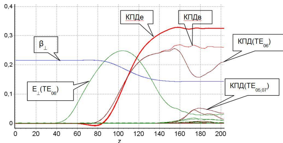
Рис. 2. Интегральные характеристики гиротрона
