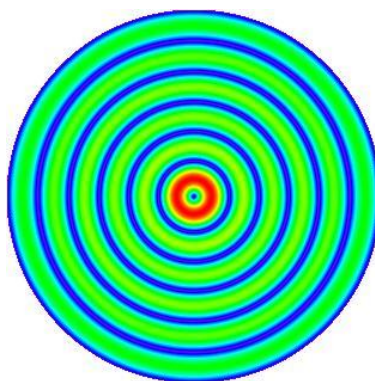
Рис. 5. Поперечное сечение модуля электрической напряженности поля в волноводе гиротрона
