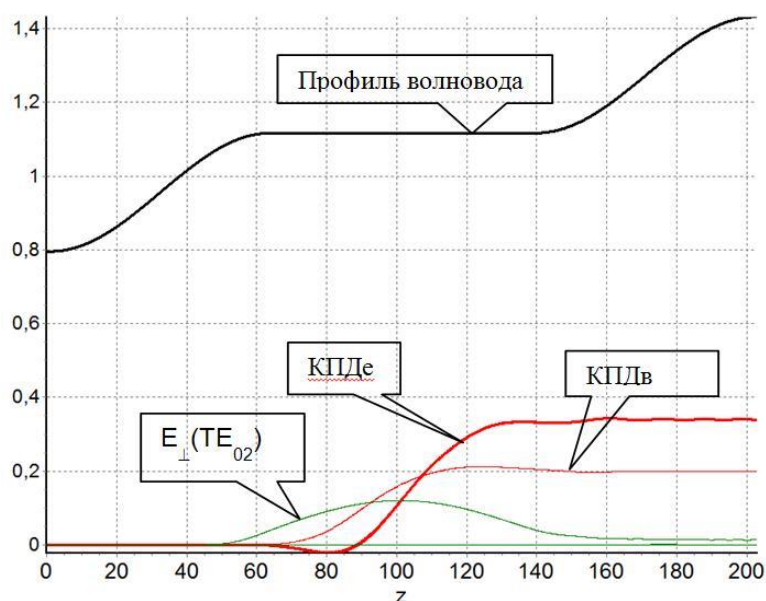
Рис. 7. Интегральные характеристики гиротрона на моде H_{02}
