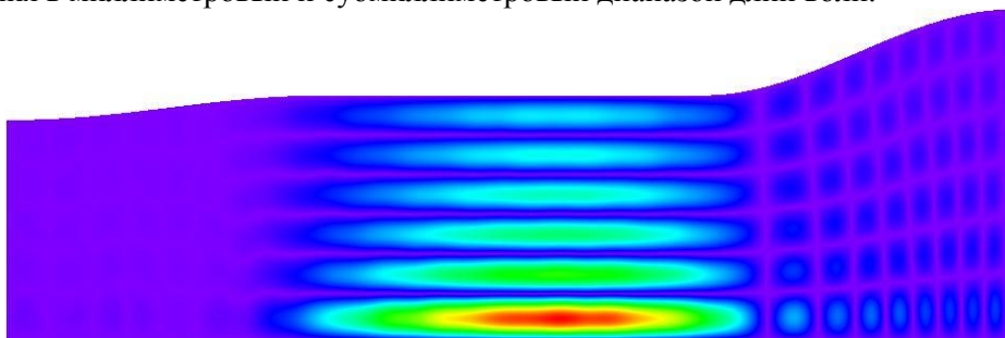
Рис. 4. Продольное сечение модуля электрической напряженности поля в волноводе гиротрона
