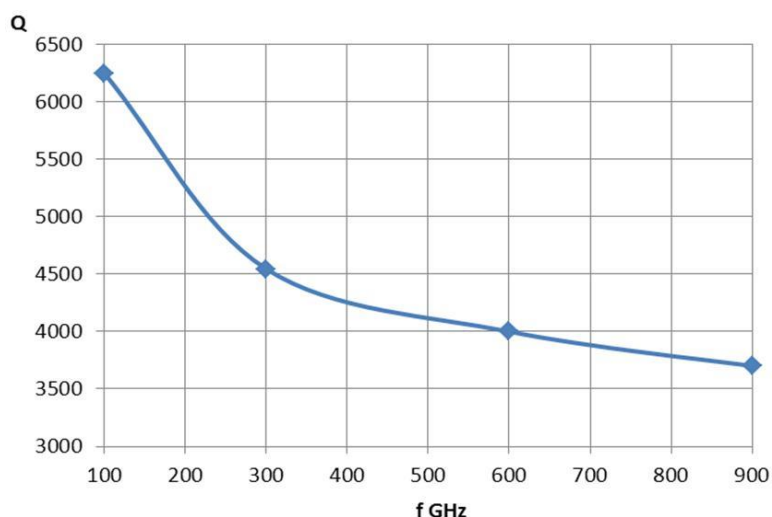
Рис. 6. Зависимость собственной добротности резонатора от частоты для волновода из меди
