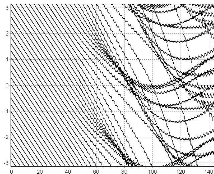
Рис. 3. Фазовые траектории электронов
