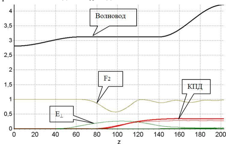
Рис. 1. Профиль волновода и основные интегральные характеристики гиротрона
