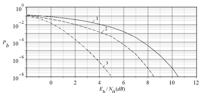
Рис. 1. Оценка характеристик кодовых конструкций в канале с АБГШ: 1 – некодированный BPSK-сигнал; 2 – (31, 6, 7)_2 Rijndael-код с ДМП; 3 – (31, 6, 15)_2 БЧХ-код с декодированием на основе алгоритма Берлекемпа-Мессис
