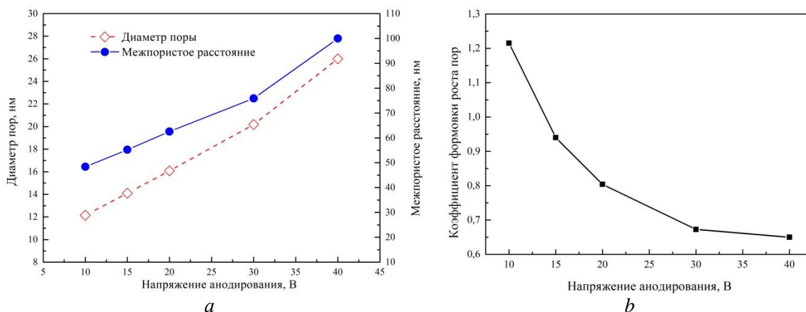
Рис. 1. Изменение диаметра пор, расстояния между центрами пор (a) и коэффициента формовки роста пор (b) с ростом напряжения анодирования Fig. 1. Change in pore diameter, the distance between the centers of the pores (a) and the molding coefficient of pore growth (b) with increasing anodizing voltage
