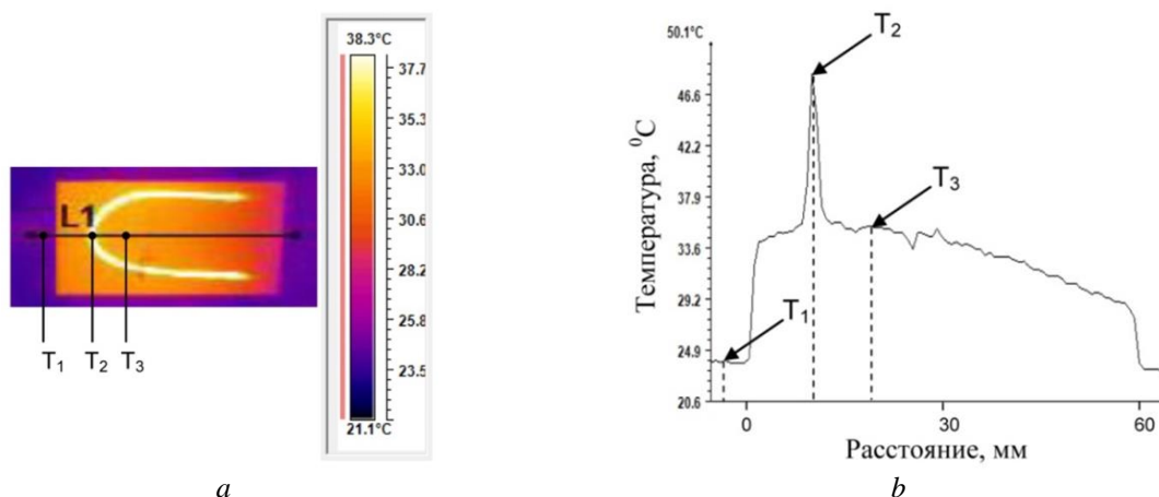
Рис. 2. Изображение платы из алюминия с слоем АОА и нагревательным элементом в тепловизионной камере (a), профиль распределения температуры через 25 с вдоль заданной линии L1 (b) с контрольными точками ( T_1 – T_3 ) при мощности нагрева 3,4 Вт: L1 – заданная линия с контрольными точками T_1 , T_2 , T_3 ; T_1 – поверхность радиатора; T_2 – углеродная нить; T_3 – поверхность платы
