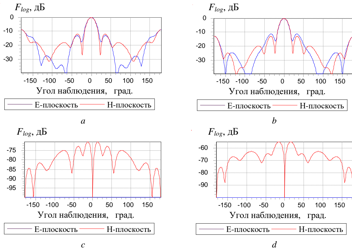
Рис. 3. Диаграмма направленности: выпуклой решетки по основной поляризации (а), плоской решетки по основной поляризации (b), выпуклой решетки с радиусами кривизны R_x = R_y = 4\lambda по кроссполаризации (c), выпуклой решетки с радиусами кривизны R_x = R_y = 2\lambda по кроссполаризации (d)
