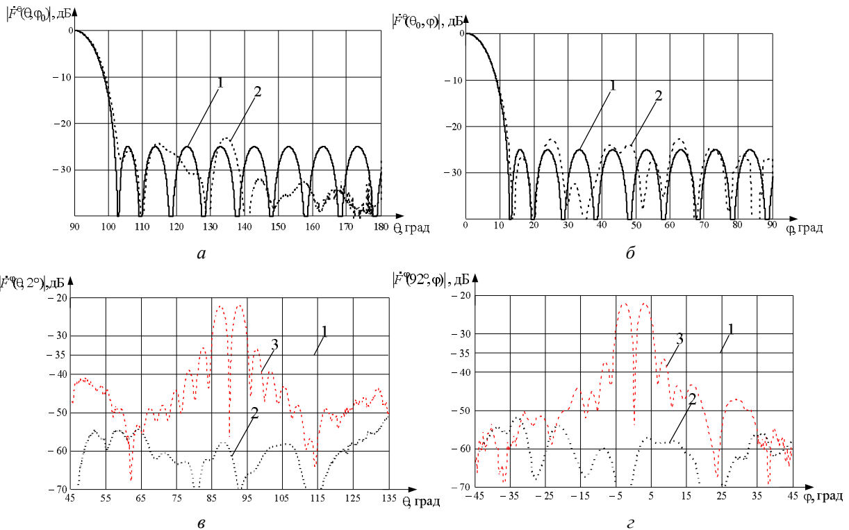
Рис. 9. Плоскостные ДН САР с заданными параметрами F_B = F_{\phi B} = F_{\theta B} = -25 дБ; 2\theta_{0,5} (2\phi_{0,5}) = 10^\circ ; K^{\text{КРОСС}} = -35 дБ: а, в – плоскость \theta F^0(\theta, \phi_0) , F^0(\theta, 2^\circ) ; б, з – плоскость \phi F^0(\theta_0, \phi) , F^0(92^\circ, \phi)
