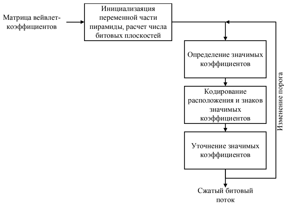
Рис. 2. Кодирование входного потока
