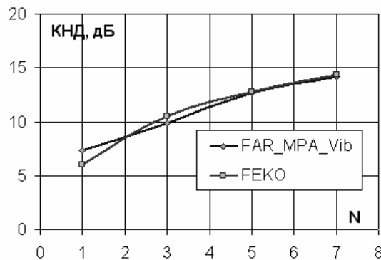
Рис. 6. Зависимость КД от количества вибраторов в антенной решетке, рассчитанная в программах FAR_MPA_Vib и FEKO
